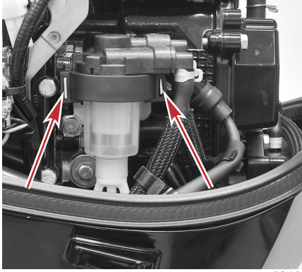
Filtre düzeneği montaj braketi
